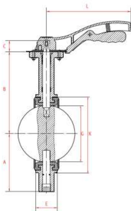
DN40-150
